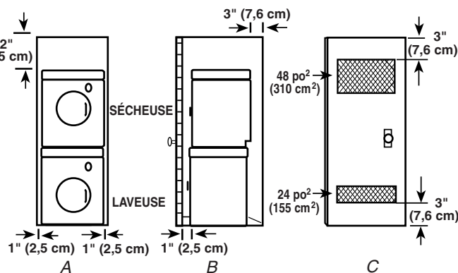
A. Encastrement B. Vue latérale - placard ou endroit exigu C. Porte de placard avec ouvertures d'entrée d'air
